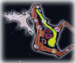
左図：カナダ/オジブア族(先住民族) に描かれた Moose (ヘラジカ) = ペガサス座の四辺形付近 (天文ソフト ステラリウムの星座絵より)
